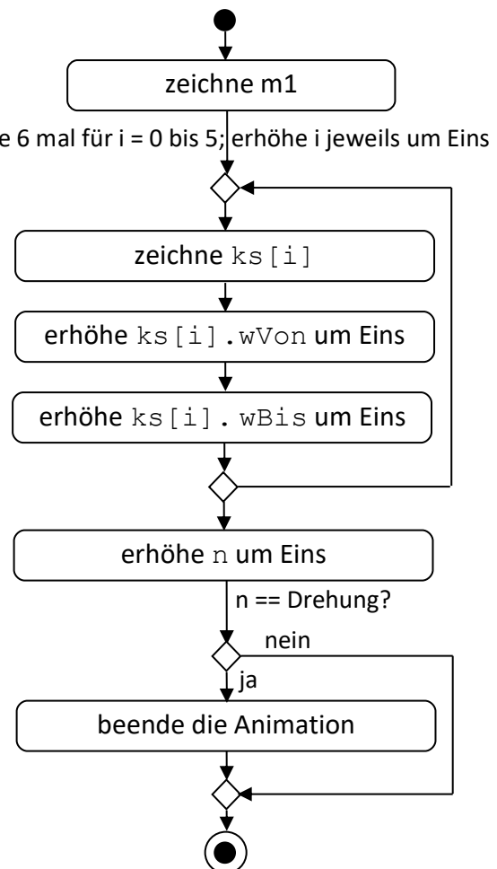
Aktivitätsdiagramm für die Methode animiere()
